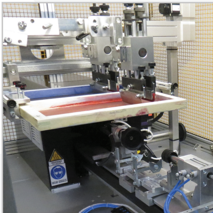
DOPPIO TELAIO DI STAMPA DOUBLE SCREEN
